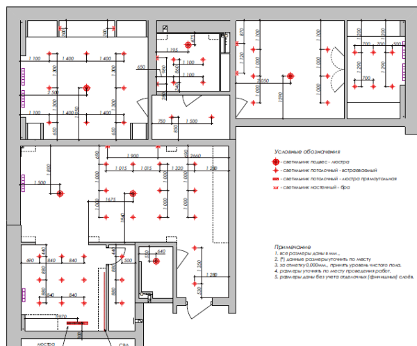
План расстановки осветительных приборов. М 1:50
