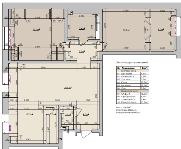
План с эргономическим анализом, М 1:50
