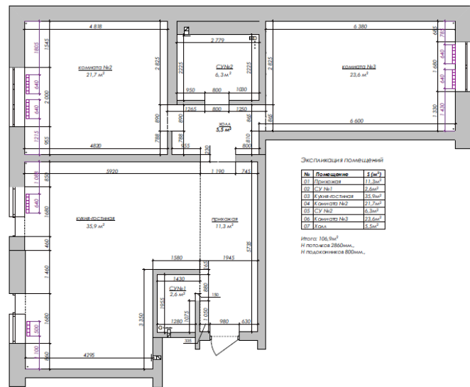
План после перепланировки М 1:50
