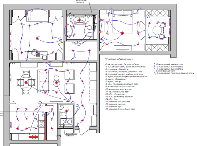
План групп выключателей. М 1:50
